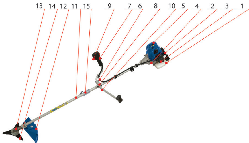
Рис. 2. Расположение основных элементов бензотриммера:
